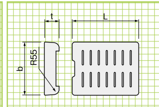
■T-2用 寸法・重量表
